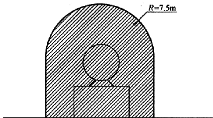
图B.0.14 露天 (棚) 设置的天然气压缩机组、阀门、法兰或类似附件的爆炸危险区域划分 距压缩机、阀门、法兰或类似附件的壳体 7.5\text{m} 以内并延至地面的空间划为 2 区。
